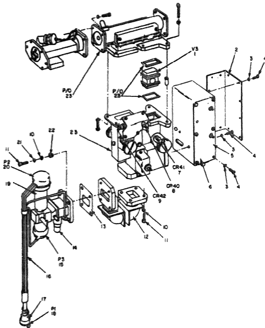
Figure 32. Mixer-Duplexer Module (1A10).
